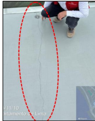
Imagen N°119: Fisuras transversales en el puente peatonal
