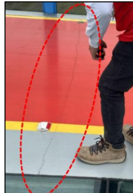
Imagen N° 120: Fisuras transversales en el puente peatonal
