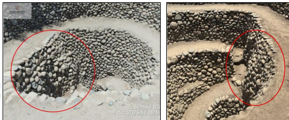
Imágenes N° 49 y 50 : Pandeamiento en el Respiradero N° 4
